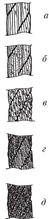
Рис. 6. Поверхностная коррозия проволок каната крестовой свивки: а — начальное окисление поверхности; б — общее окисление поверхности; в — заметное окисление; г — сильное окисление; д — интенсивная коррозия
