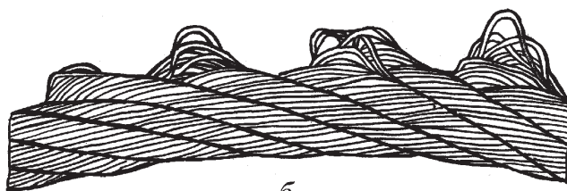
Рис. 12. Выдавливание проволок прядей: а — в одной пряди; б — в нескольких прядях
