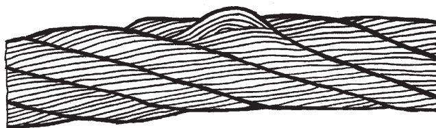
Рис. 11. Выдавливание сердечника
