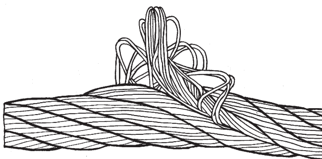
Рис. 11. Выдавливание сердечника
