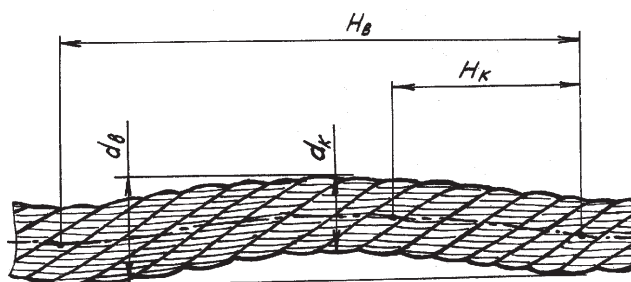
Рис. 9. Волнистость каната (объяснение в тексте)
